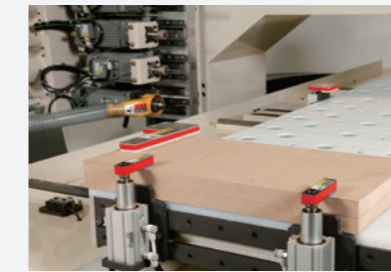
フロア吸着+上クランプ押え（標準装備）
